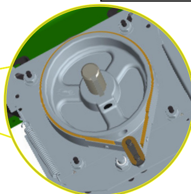
Détail du frein solénoïde
