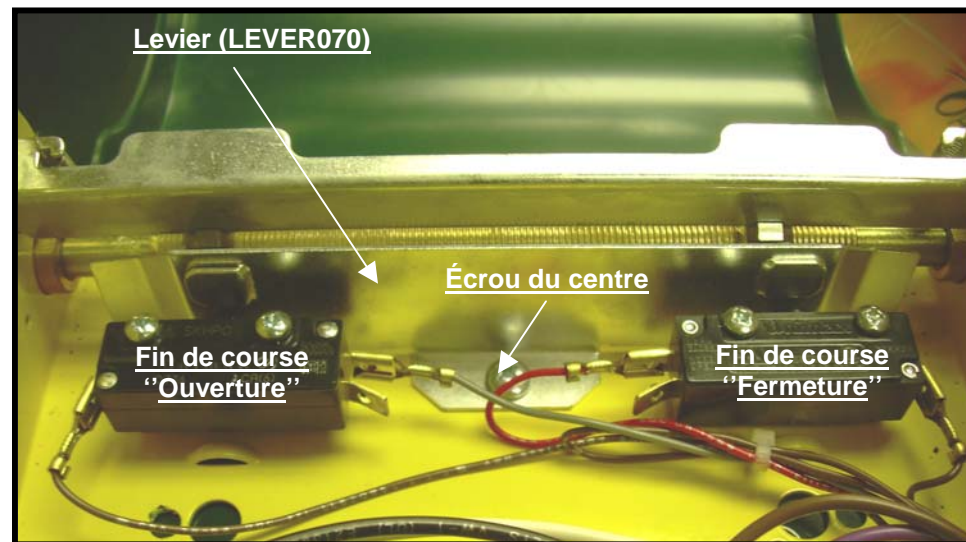
Représentation d'une boîte de contrôle "Opera" avec l'ancien système de fin de course.
