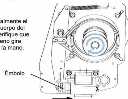
Figura 46 - Procedimiento de ajuste de la banda de freno
