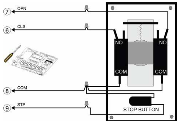
Figura 40 - KEYSWITCH 019 (interruptor de llave)
