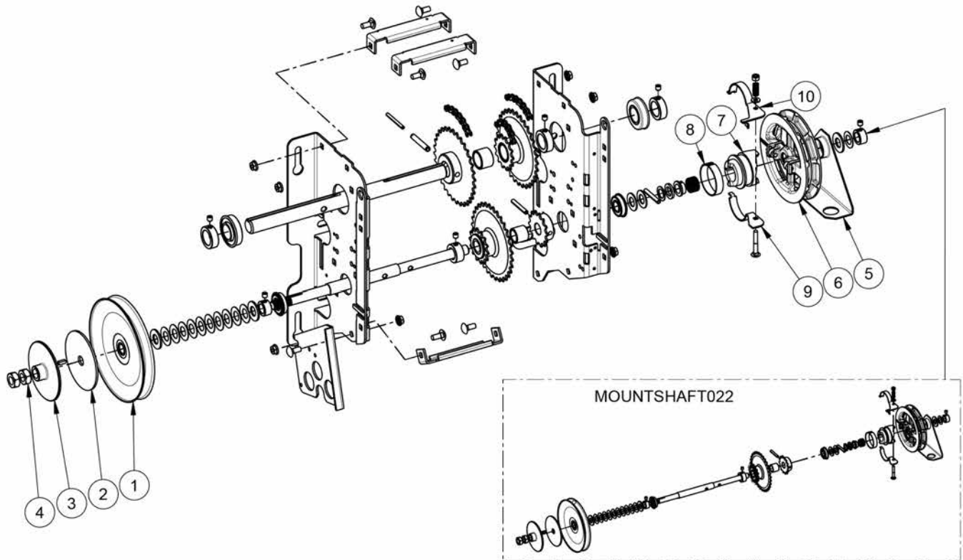
Figure 5 - Despiece Mecánico Opera-MH
