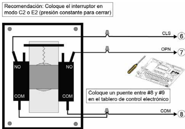
Figura 39 - KEYSWITCH 010 / 015 (interruptor de llave)
