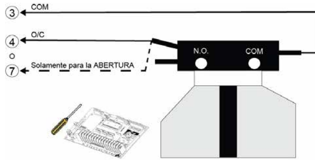
Figura 38 - PULLCORD 001 / 003 / 004 / 007 (cordón de tiro)
