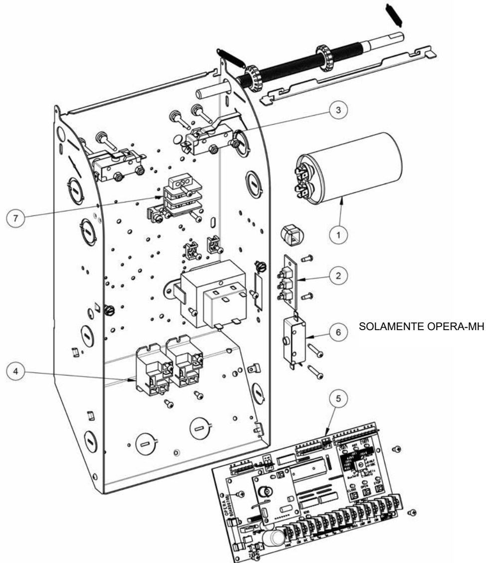
Figure 7 - Caja de Control Opera-MH, Opera-MJ y OMT con Tablero de Control 070M
