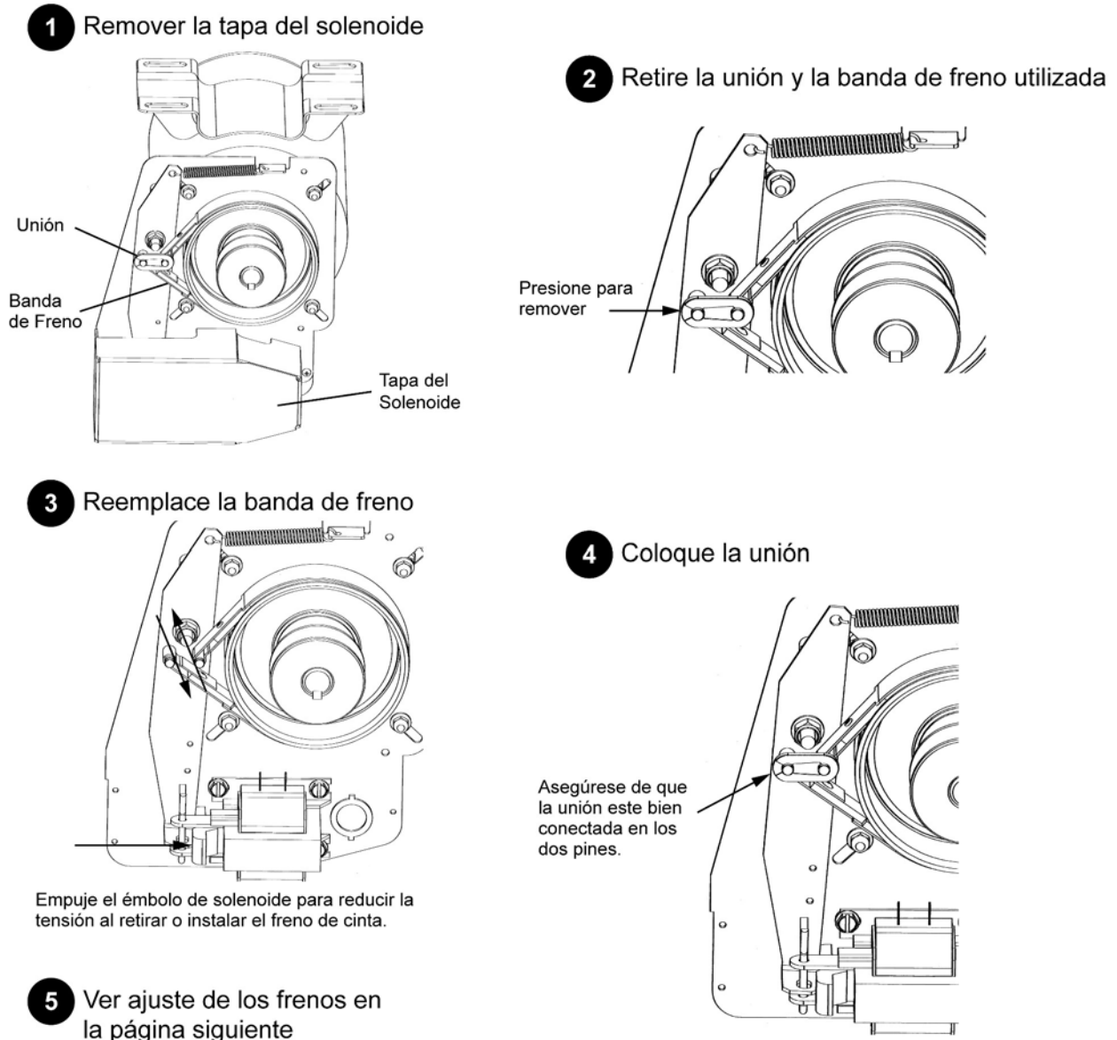
Figura 45 - Procedimiento de reemplazo de la banda de freno
