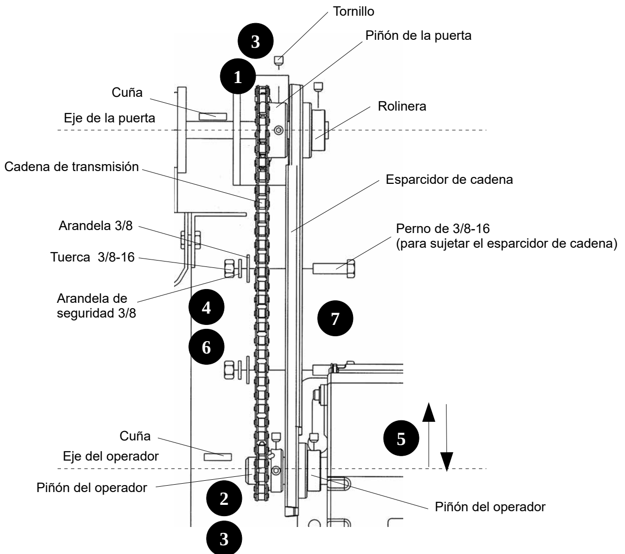
Figura 7 - Componentes Hardware
