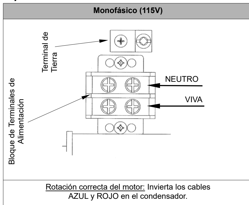
Figura 15 - Conexiones de bajo voltaje (control) y alto voltaje (alimentación)
