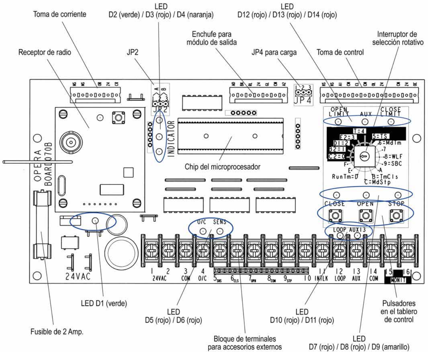
Figura 42 - Tablero de control electrónico – BOARD 070M
