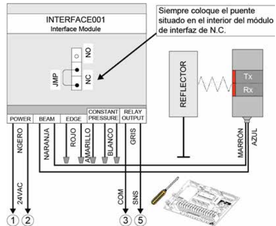
Figura 29 - PHOTO 008D1 / D2 (Foto celdas)
