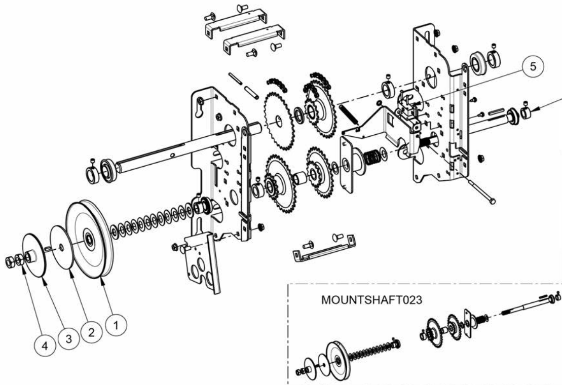
Figure 6 - Despiece Mecánico Opera-MJ
