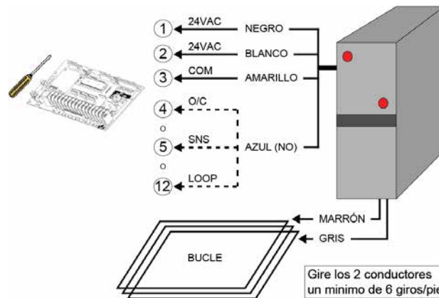
Figura 41 - Detector de bucle de inducción
