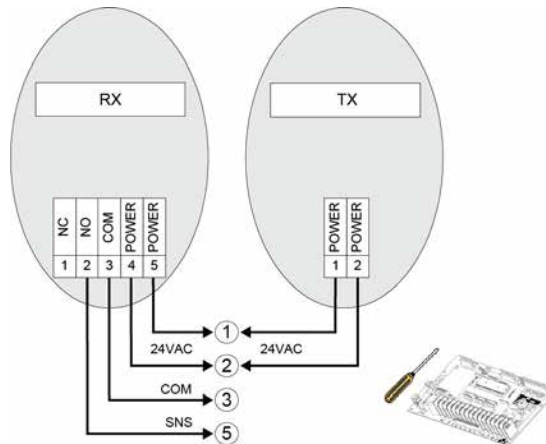
Figura 30 - PHOTO 015 / 016 / 045 / 050 / 051 / 059 (Foto celdas)
