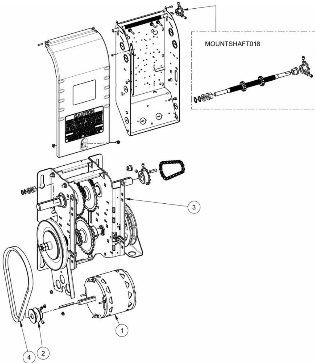
Figura 4 - Despiece Mecánico Opera-MH & Opera-MJ
