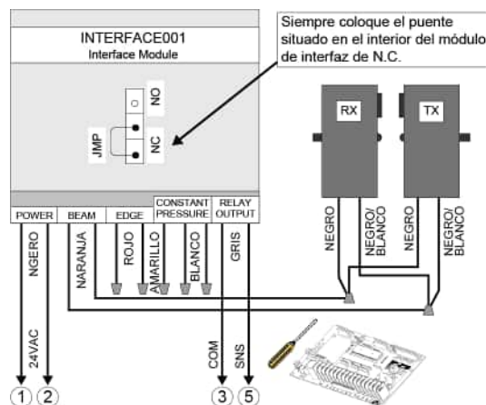
Figura 30 - PHOTO 008C3 / C4 / E1 (celdas fotoeléctricas)
