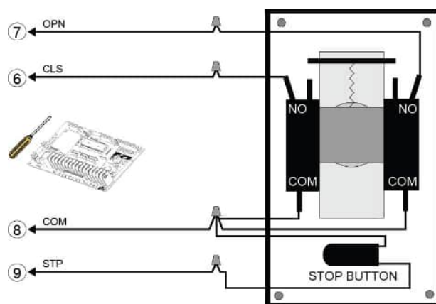
Figura 42 - KEYSWITCH 019 (Interruptor de llave)
