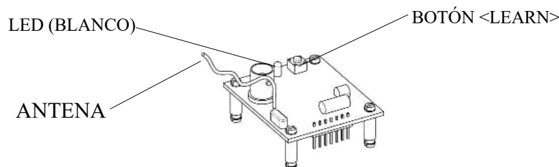
Figura 45 - RADIORE100 (ECB BOARD 070)
