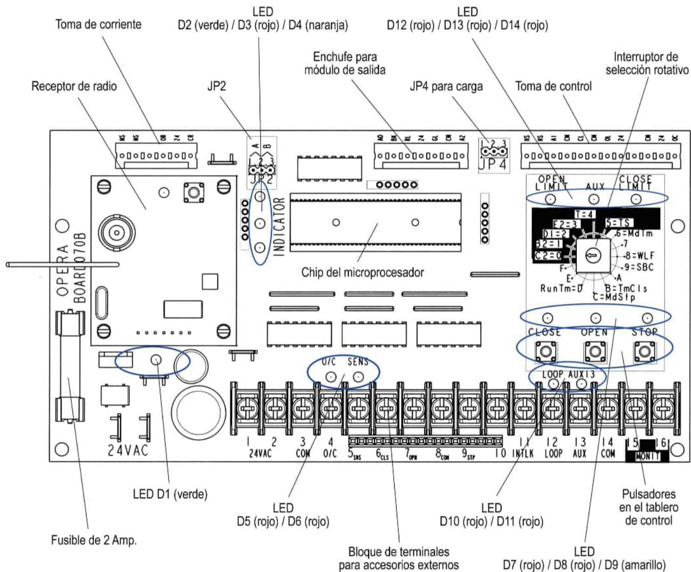
Figura 44 - Tablero de control electrónico – BOARD 070M
