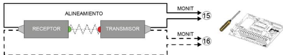
Figura 27 - SENSEEDGE042 instalación
