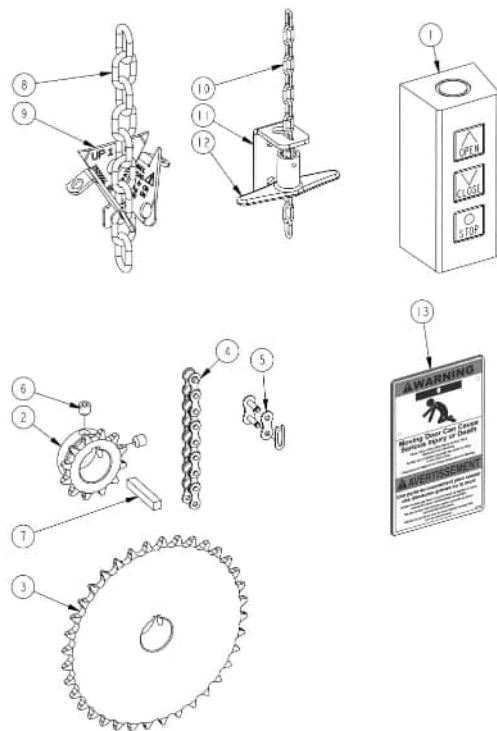
Figura 4 - Hardware para eje de transmisión estándar
