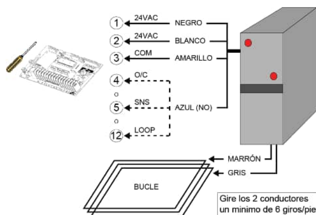
Figura 43 - Detector de bucle de vehículo
