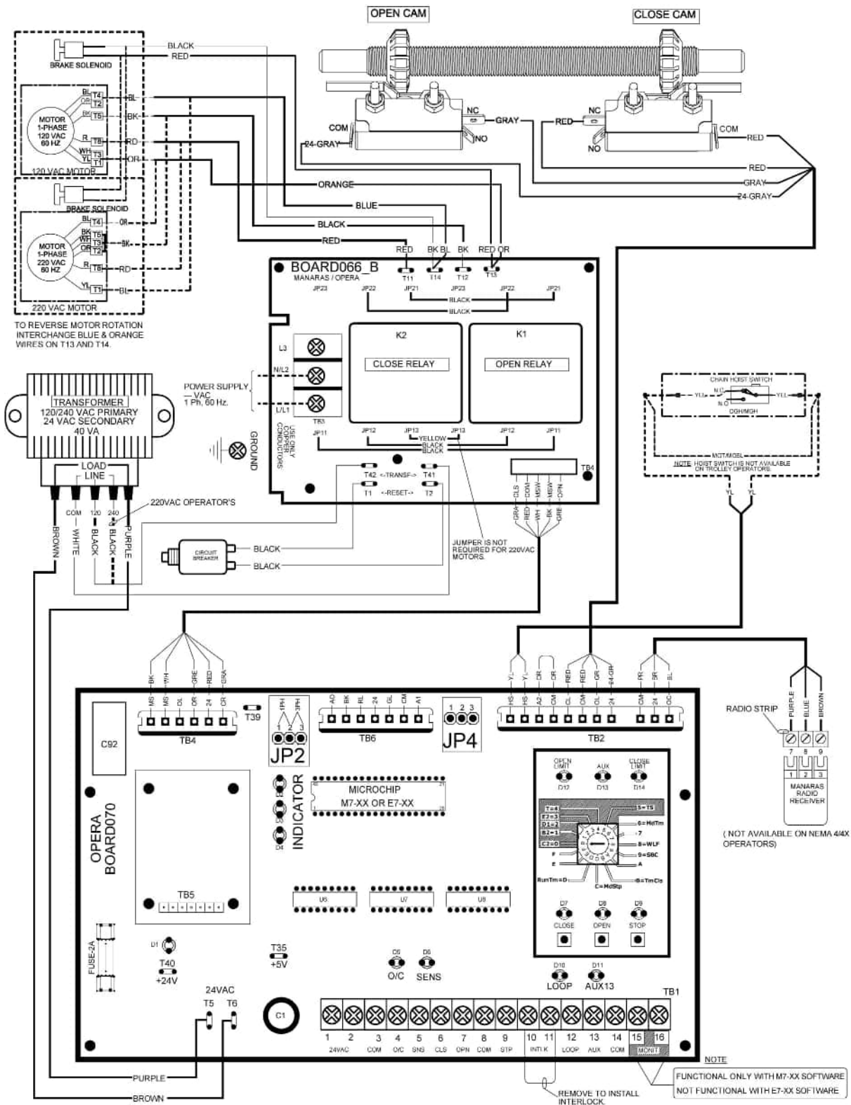
Figura 51 - EDWG1107006602
