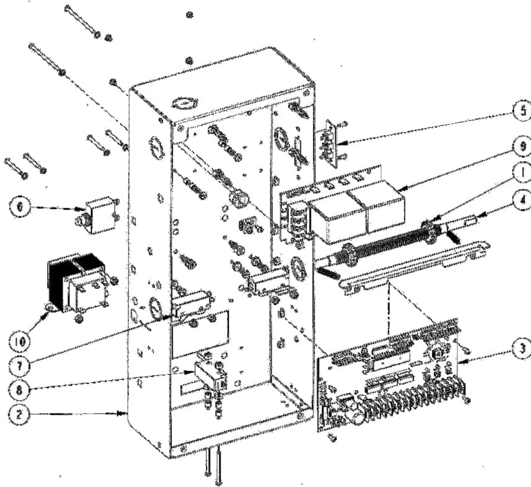
Figura 58 - Caja de control MGH y MRGH con tablero de control electrónico BOARD 070M
