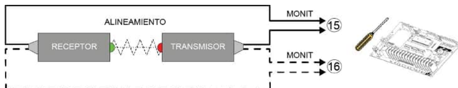
Figura 24 - PHOTO 061 / 061A / 070 instalación
