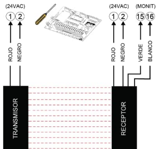
Figura 28 - LIGHTCURTAIN 001 / 002 instalación
