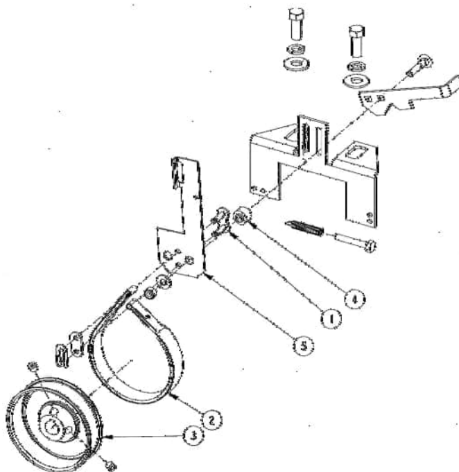
Figura 57 - Despiece mecánico de BRAKE 012
