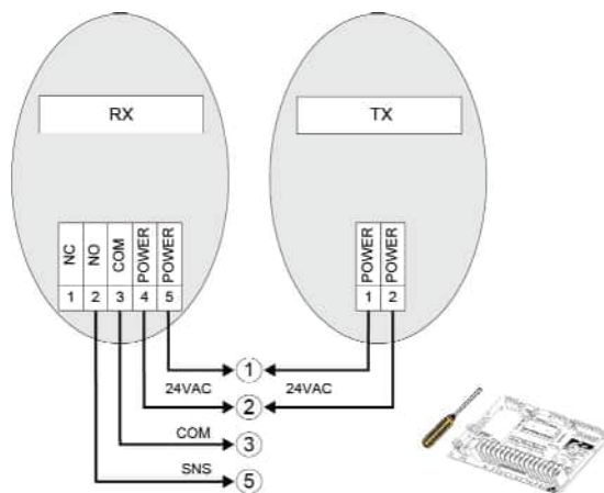
Figura 32 - PHOTO 015 / 016 / 045 / 050 / 051 / 059 (celdas fotoeléctricas)
