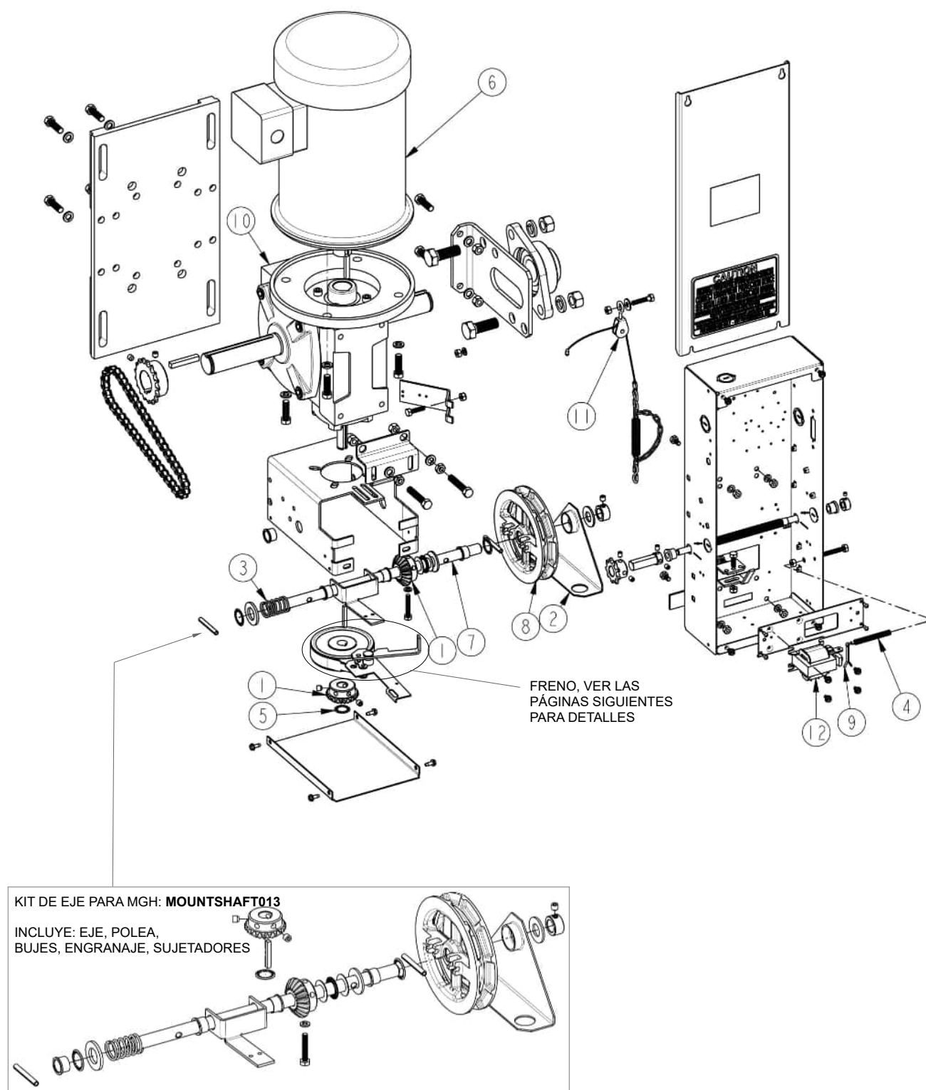
Figura 56 - Despiece mecánico MRGH (2, 3, 5 HP) Componentes de repuesto, ver la Tabla 17, p.56
