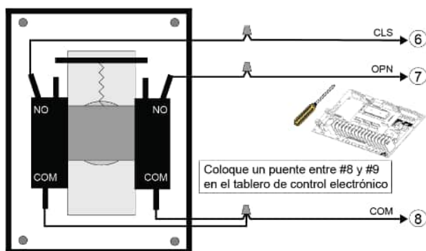
Figura 41 - KEYSWITCH 010 / 015 (Interruptor de llave)
