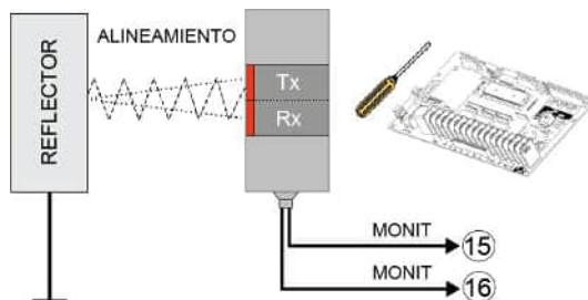
Figura 25 - Instalación de PHOTO 065
