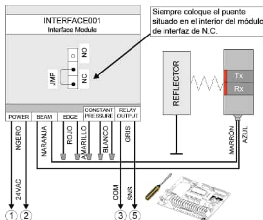
Figura 31 - PHOTO 008D1 / D2 (celdas fotoeléctricas)
