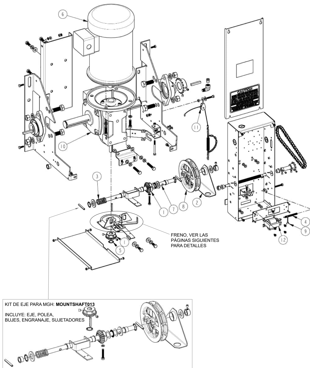
Figura 55 - Despiece mecánico MGH (2, 3, 5 HP) Componentes de repuesto, ver la Tabla 17, p.56
