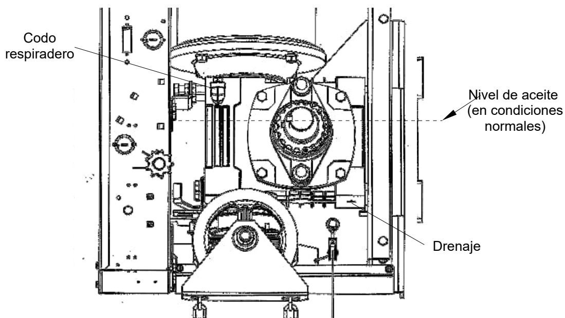
Figura 50 - Respiradero del reductor de engranajes
