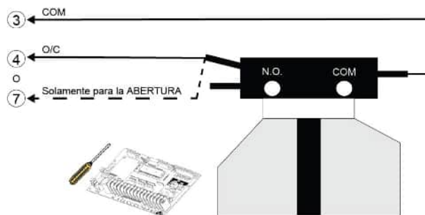
Figura 40 - PULLCORD 001 / 003 / 004 / 007 (cordón de tiro)
