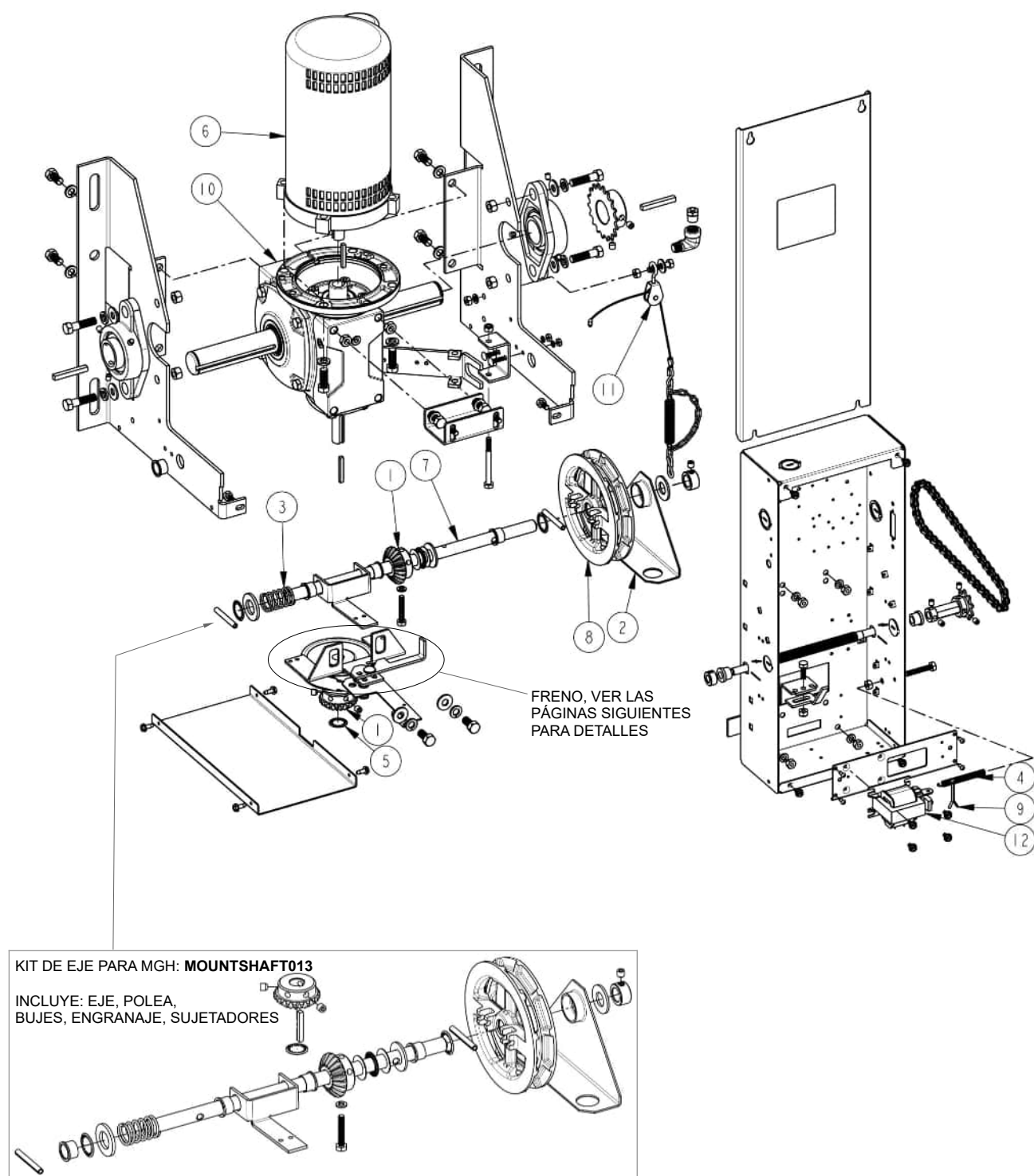
Figura 54 - Despiece mecánico MGH (½, ¾, 1, 1-½ HP) Componentes de repuesto, ver la Tabla 17, p.56
