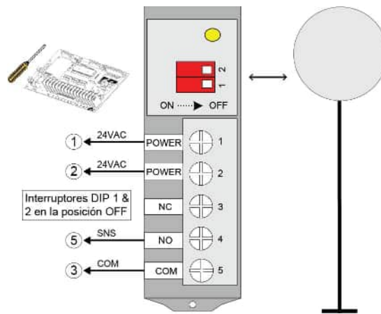
Figura 33 - PHOTO 060 (celdas fotoeléctricas)
