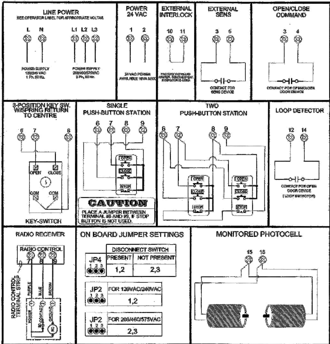
Figura 53 - External Wiring
