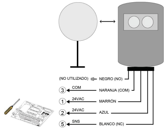
Figura 25 - PHOTO 038 (celdas fotoeléctricas)
