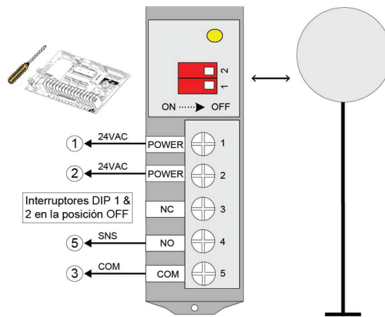
Figura 23 - PHOTO 060 (celdas fotoeléctricas)
