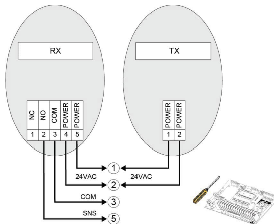
Figura 22 - PHOTO 015 / 016 / 045 / 050 / 051 / 059 (celdas fotoeléctricas)
