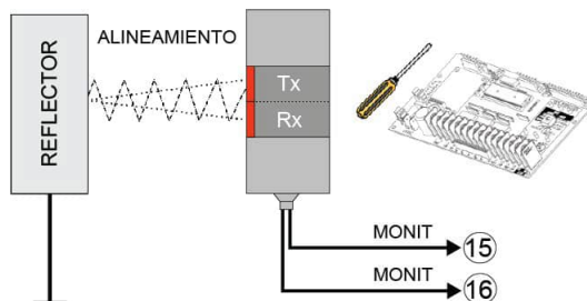
Figura 15 - Instalación de PHOTO 065
