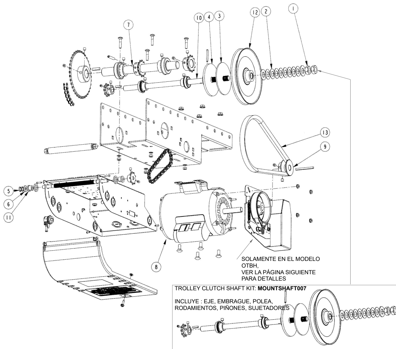
Figura 42 - Despiece mecánico OTH / OTBH
