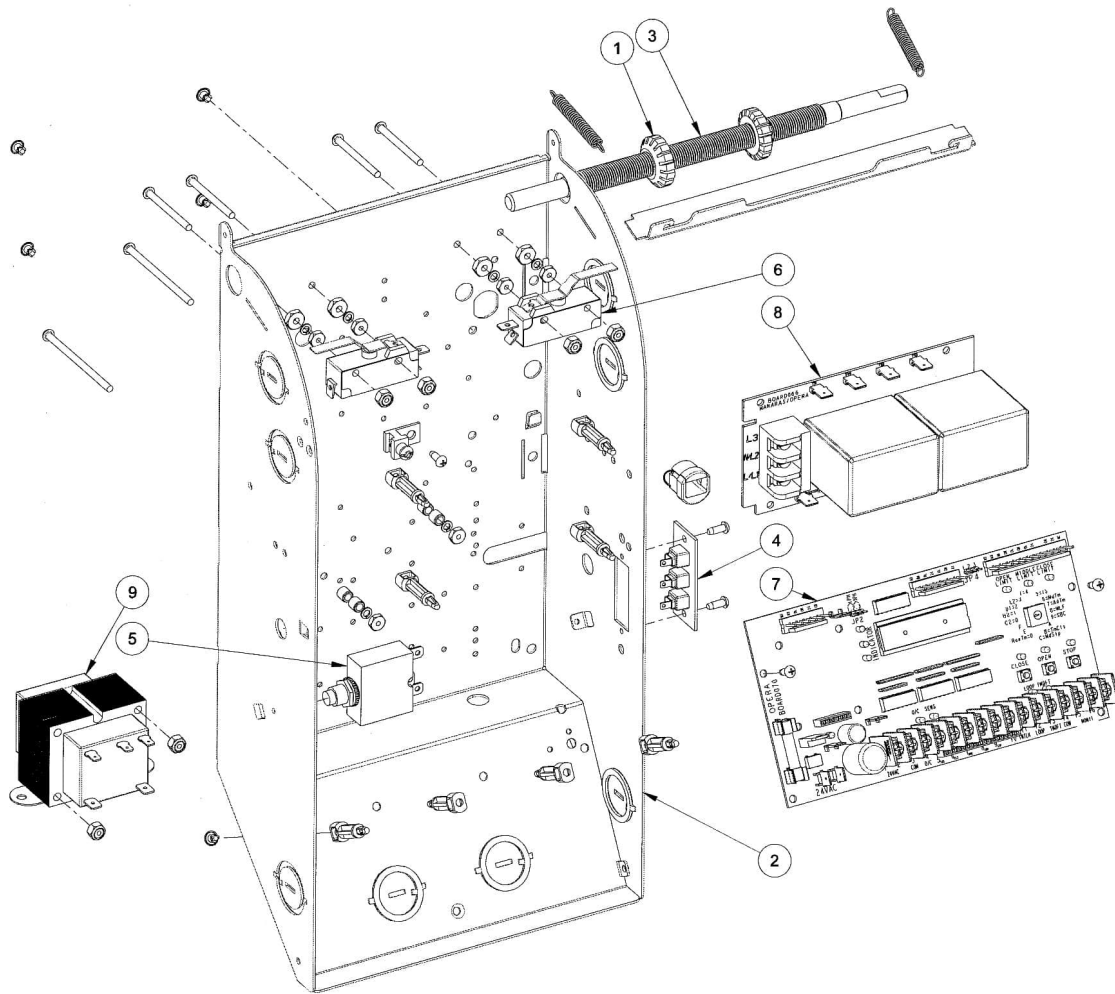
Figura 44 - Caja de control OTH / OTBH / MGT con tablero de control electrónico BOARD 070M
