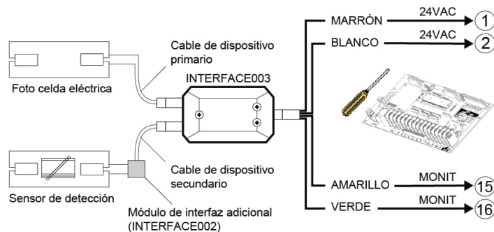
Figura 19 - INTERFACE 003 instalación
