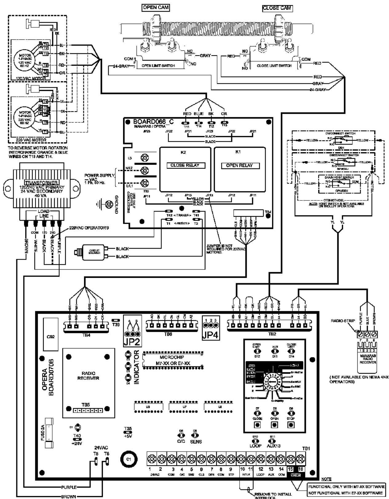
Figura 39 - EDWG1107006601
