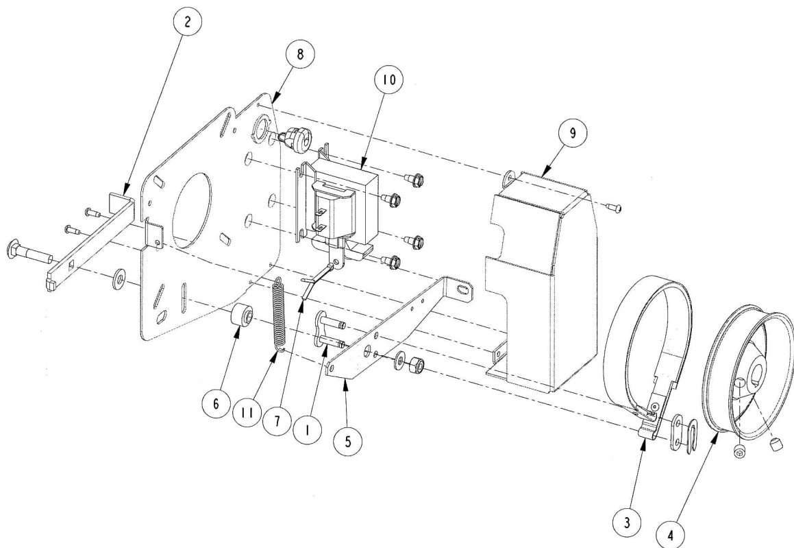
Figura 43 - Despiece mecánico de BRAKE 011
