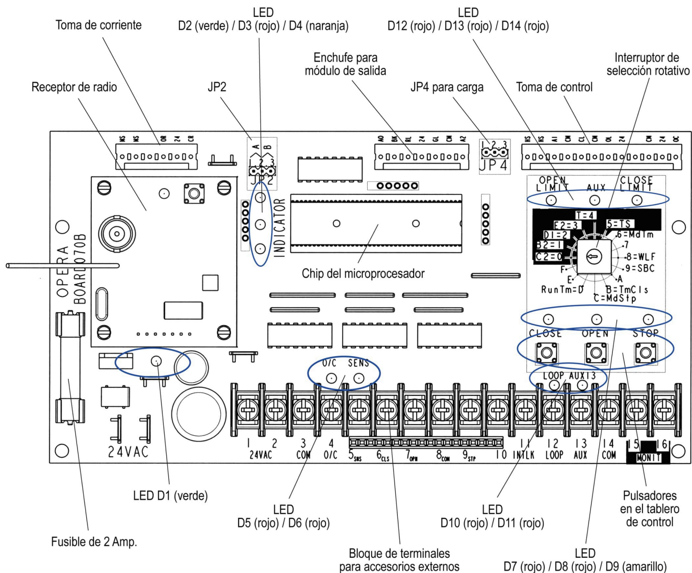
Figura 34 - Tablero de control electrónico – BOARD 070M
