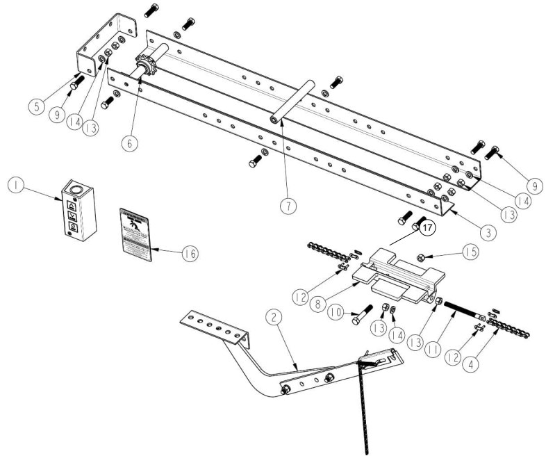
Figura 3 - Hardware estándar de operador tipo trole
