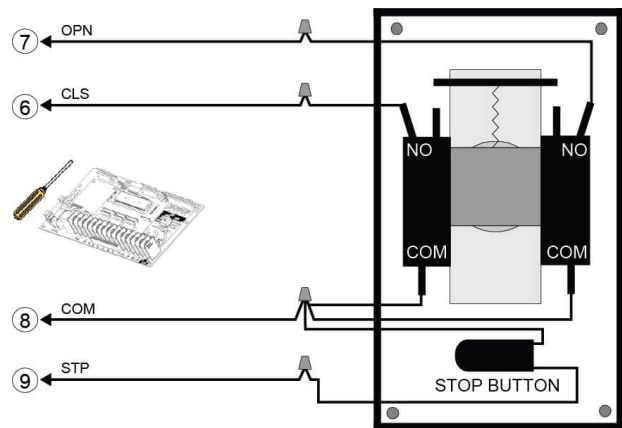
Figura 32 - KEYSWITCH 019 (Interruptor de llave)
