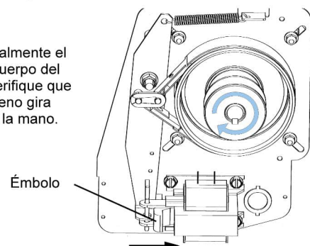
Figura 38 - Procedimiento de ajuste de la banda de freno
