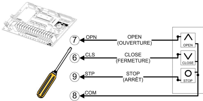
Figura 8 - STATION 020 / 084 (estación) 3-PBS Abrir / Cerrar / Detener
