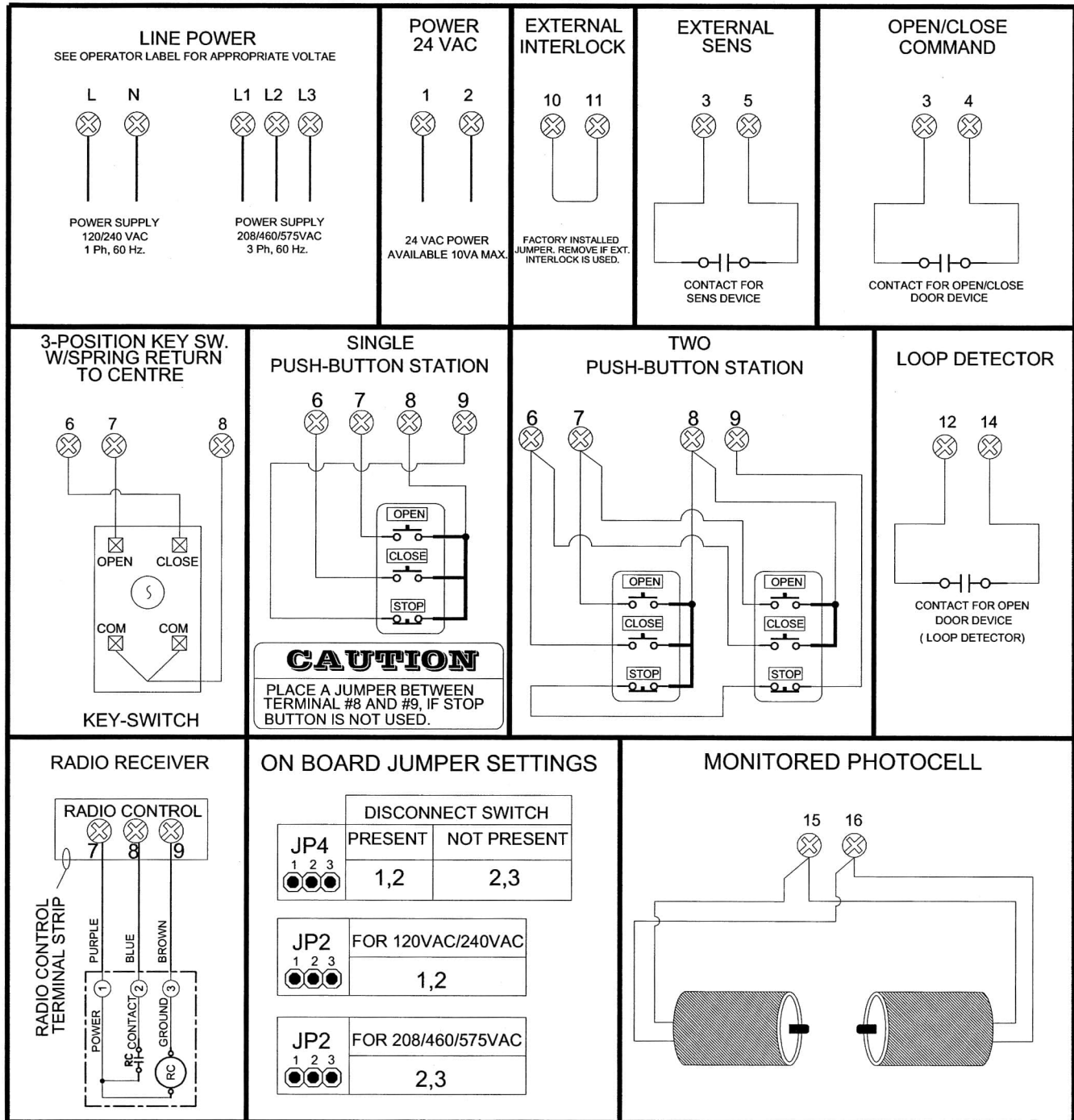
Figura 41 - Cableado externo
