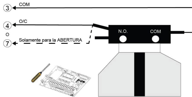
Figura 30 - PULLCORD 001 / 003 / 004 / 007 (cordón de tiro)
