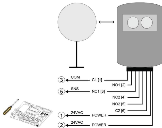
Figura 24 - PHOTO 018 (celdas fotoeléctricas)
