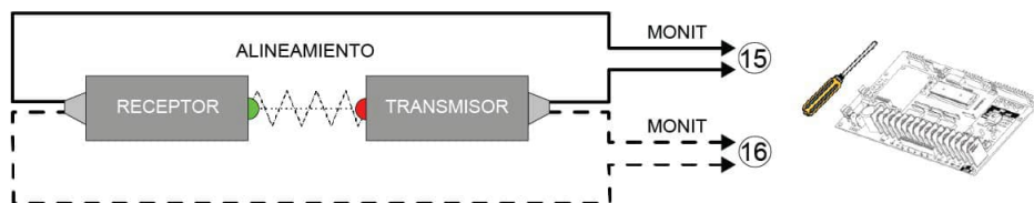
Figura 14 - PHOTO 061 / 061A / 070 instalación
