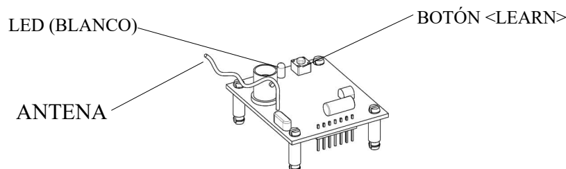
Figura 35 - RADIORE100 (ECB BOARD 070)
