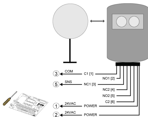
Figura 23 - PHOTO 018 (celdas fotoeléctricas)
