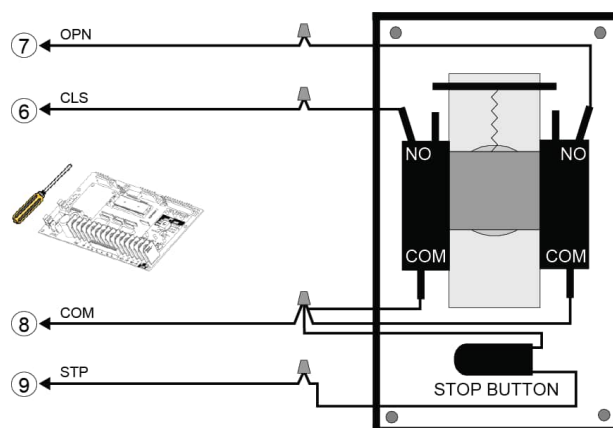
Figura 31 - KEYSWITCH 019 (Interruptor de llave)
