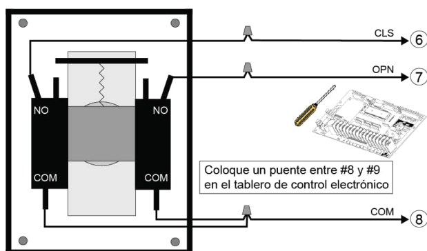
Figura 30 - KEYSWITCH 010 / 015 (Interruptor de llave)
