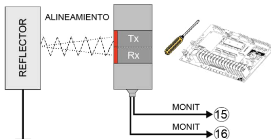
Figura 14 - Instalación de PHOTO 065
