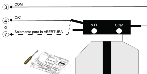
Figura 29 - PULLCORD 001 / 003 / 004 / 007 (cordón de tiro)
