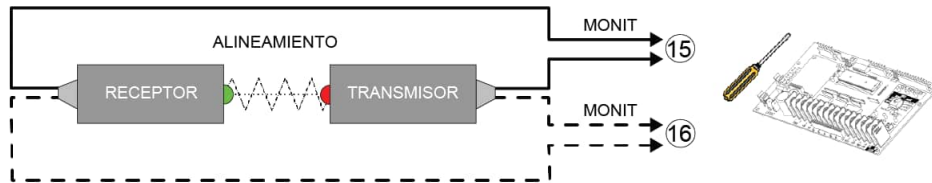
Figura 16 - SENSEEDGE042 instalación
