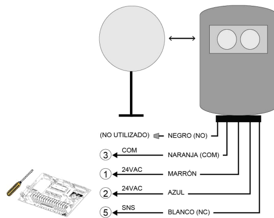
Figura 24 - PHOTO 038 (celdas fotoeléctricas)
