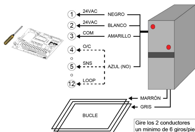
Figura 32 - Detector de bucle de vehículo
