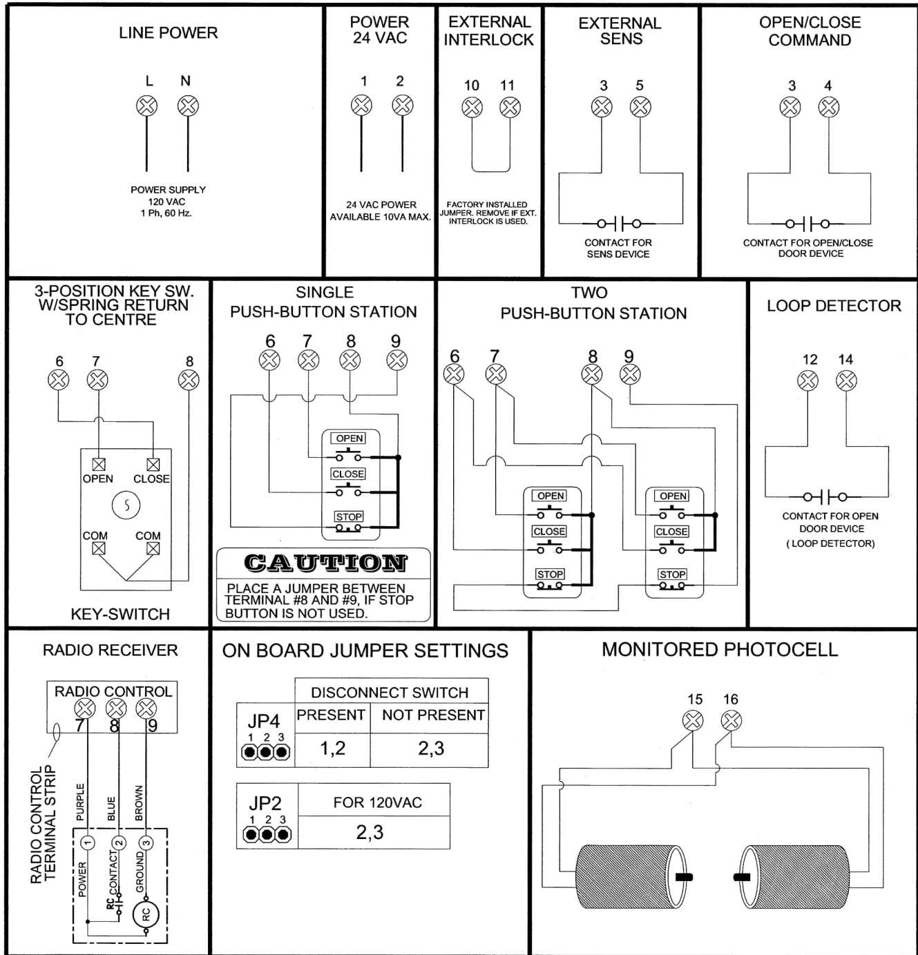
Figura 3 - Cableado externo
