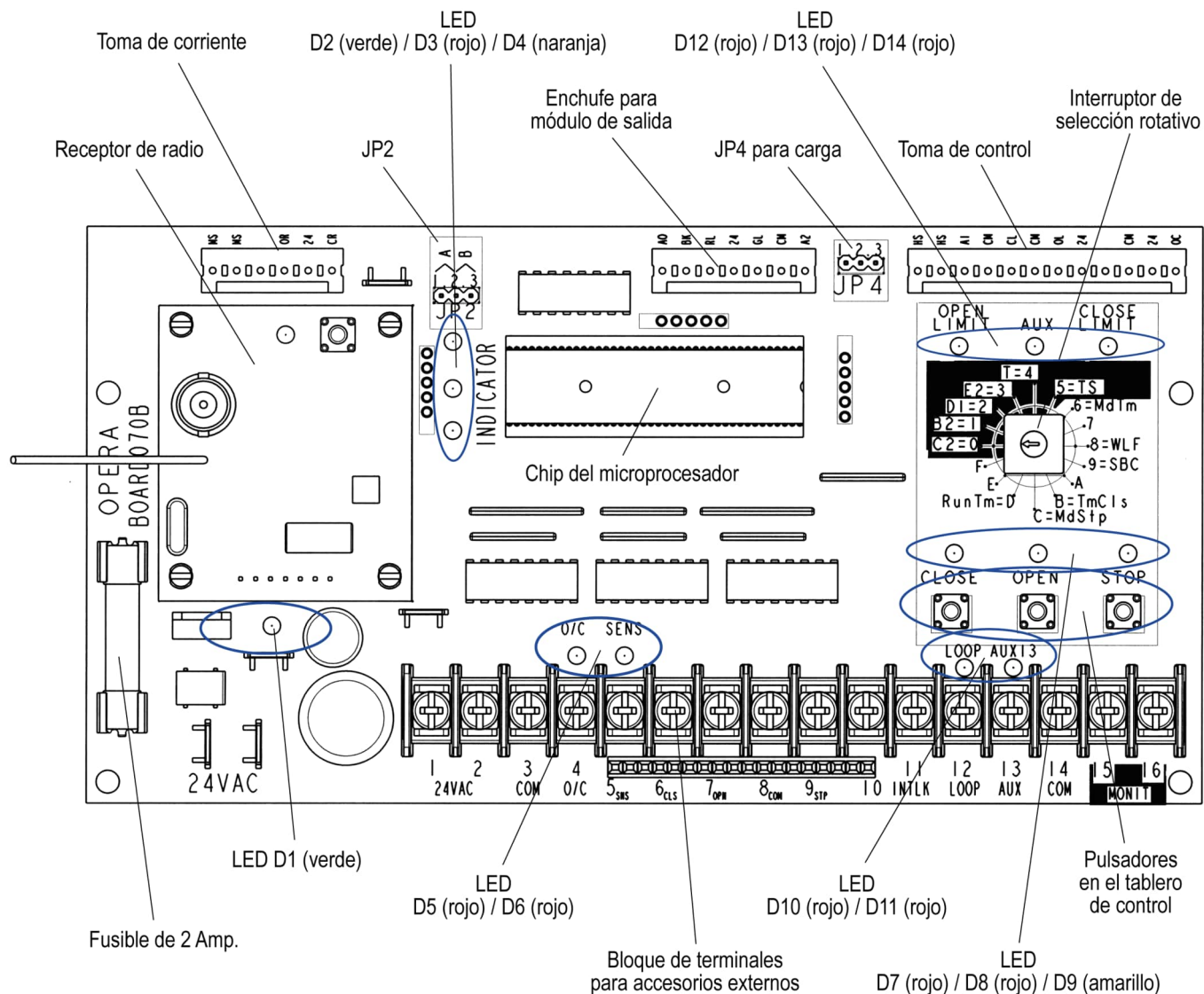
Figura 33 - Tablero de control electrónico – BOARD 070M
