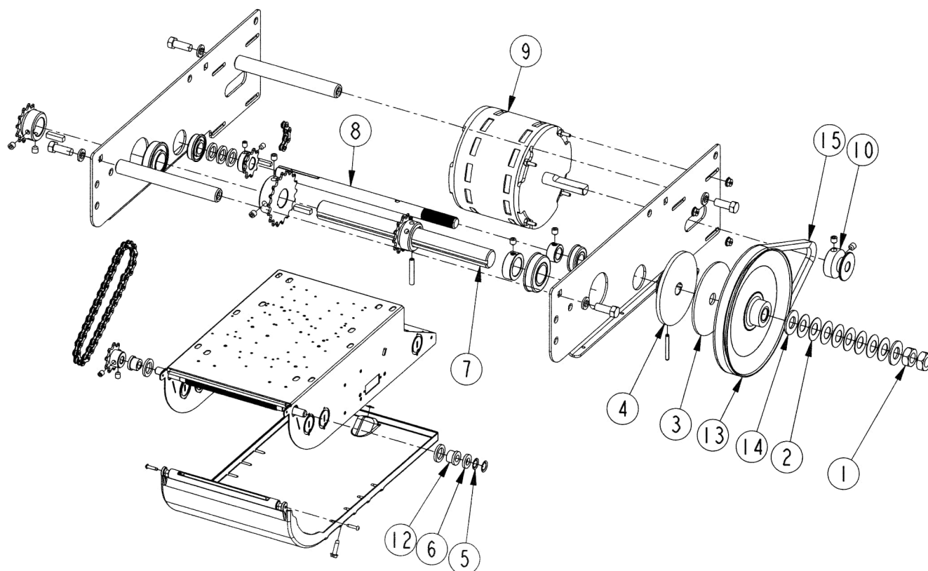
Figura 36 - Despiece mecánico OMT
