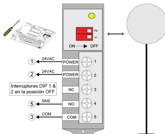
Figura 22 - PHOTO 060 (celdas fotoeléctricas)
