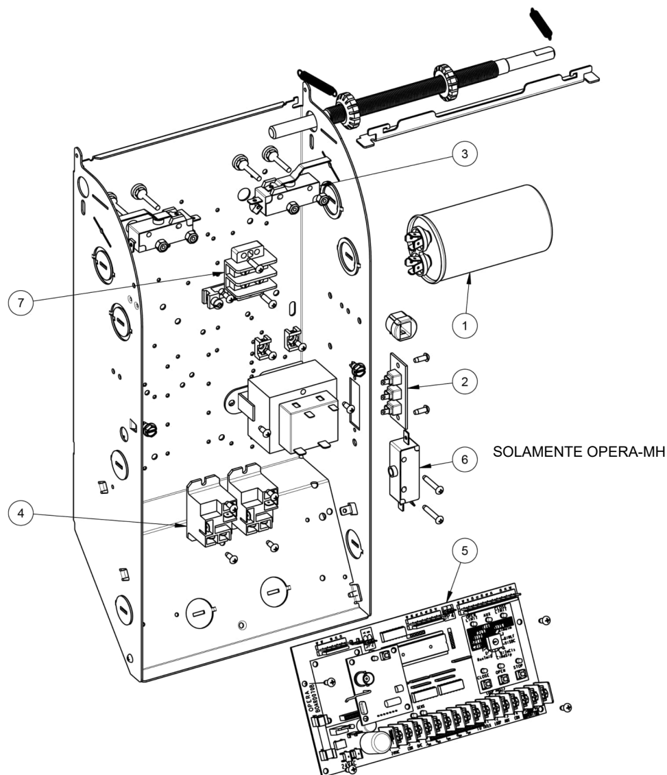
Figure 4 - Caja de control Opera-MH, Opera-MJ y OMT con tablero de control BOARD070M
