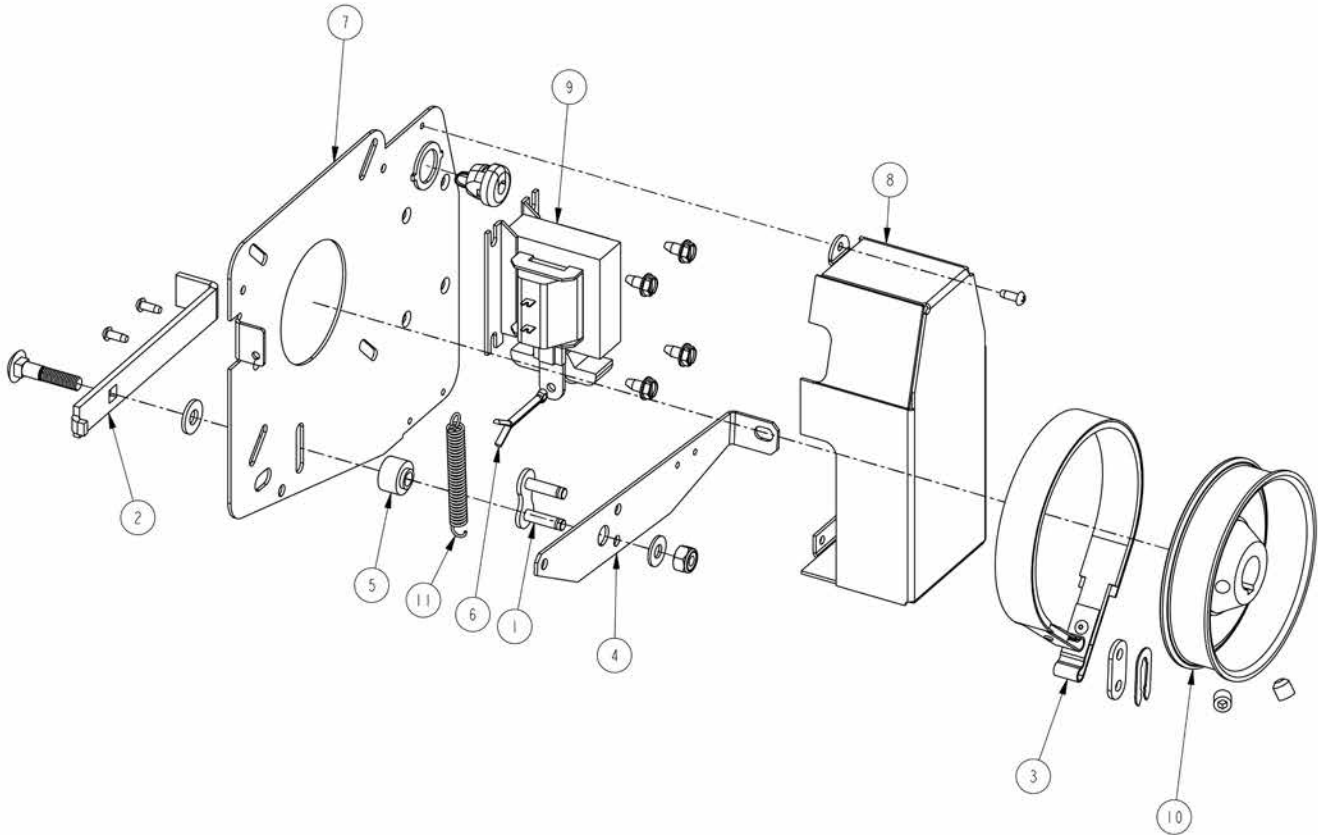
Figura 52 - Despiece mecánico BRAKE 013
