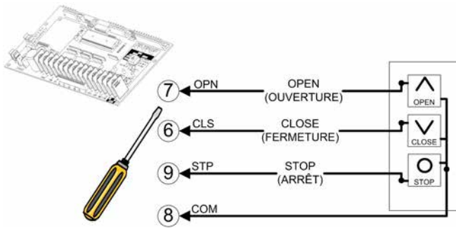
Figura 19 - STATION 020 / 084 (estación) 3-PBS Abrir / Cerrar / Detener
