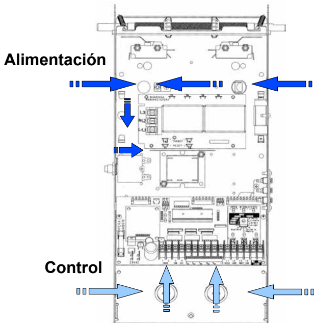
Figura 18 - Conexiones de bajo voltaje (control) y alto voltaje (alimentación)
