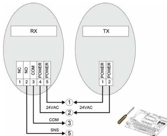
Figura 27 - PHOTO 015 / 016 / 045 / 050 / 051 / 059 (Foto celdas)
