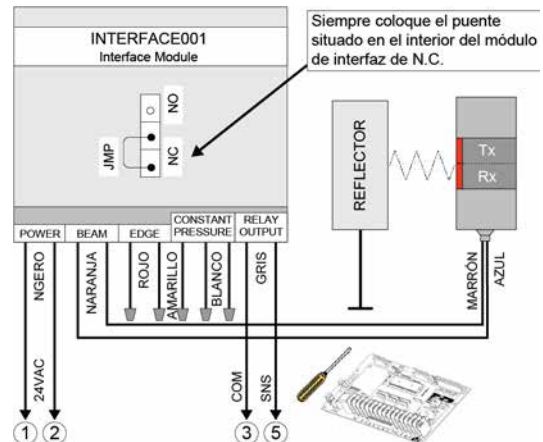
Figura 26 - PHOTO 008D1 / D2 (Foto celdas)
