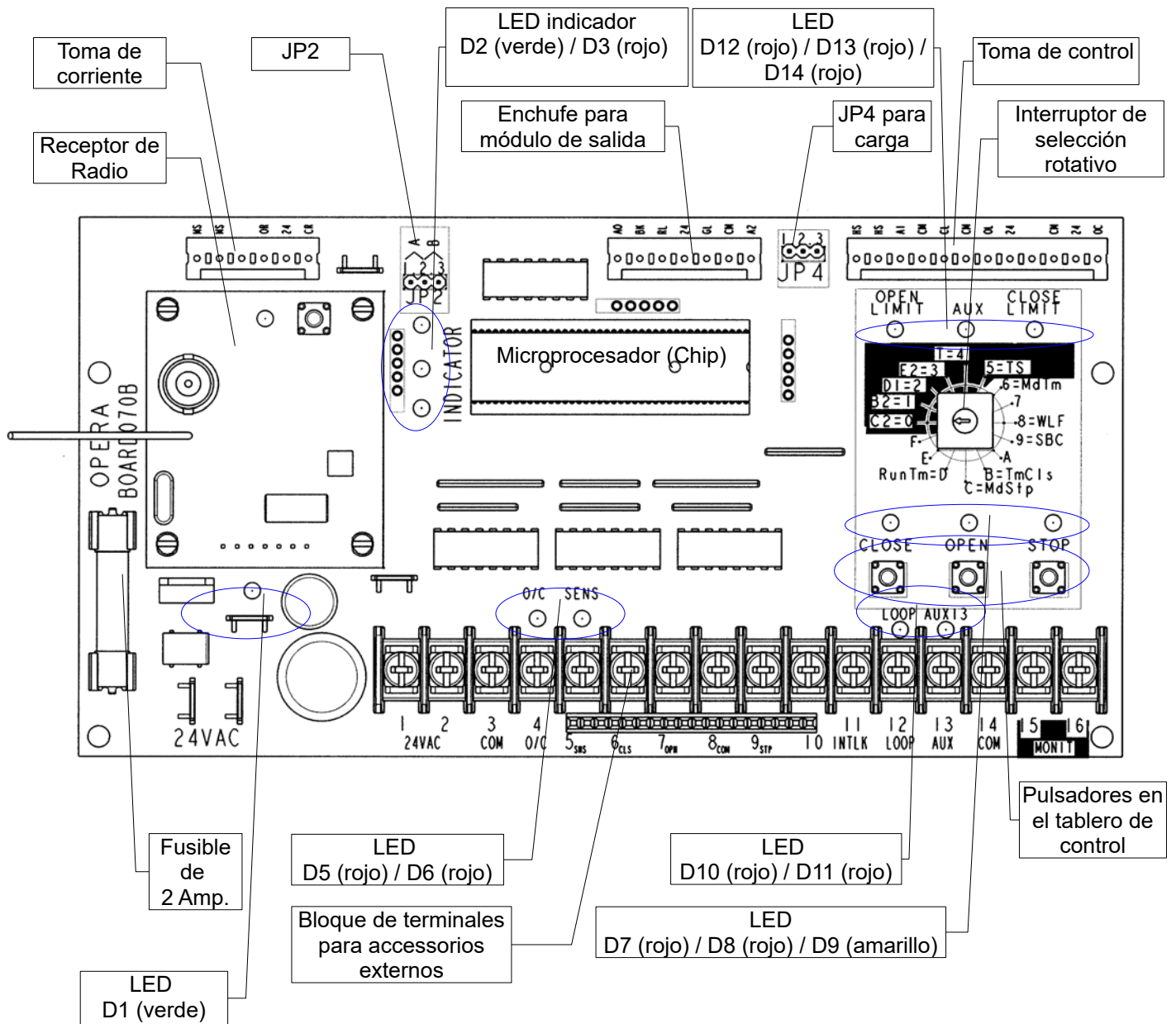
Figura 39 - Tablero de control electrónico – BOARD 070E
