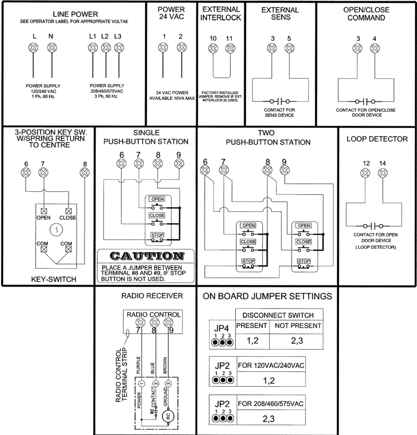
Figura 46 - Cableado externo
