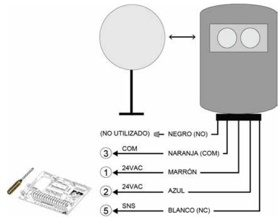
Figura 30 - PHOTO 038 (Foto Celdas)
