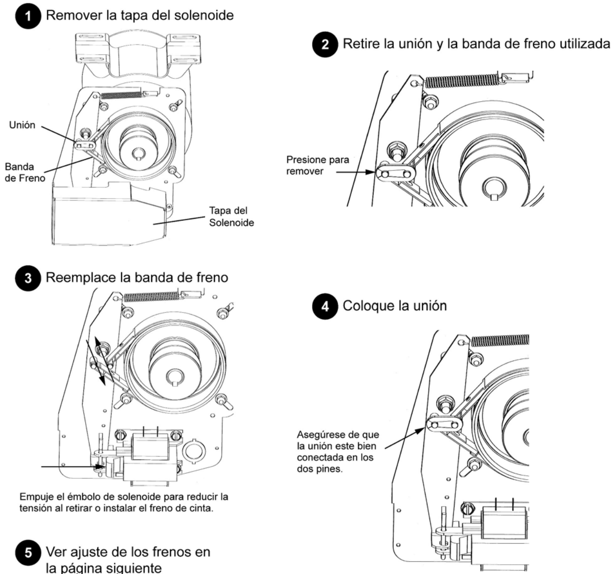
Figura 42 - Procedimiento de reemplazo de la banda de freno
