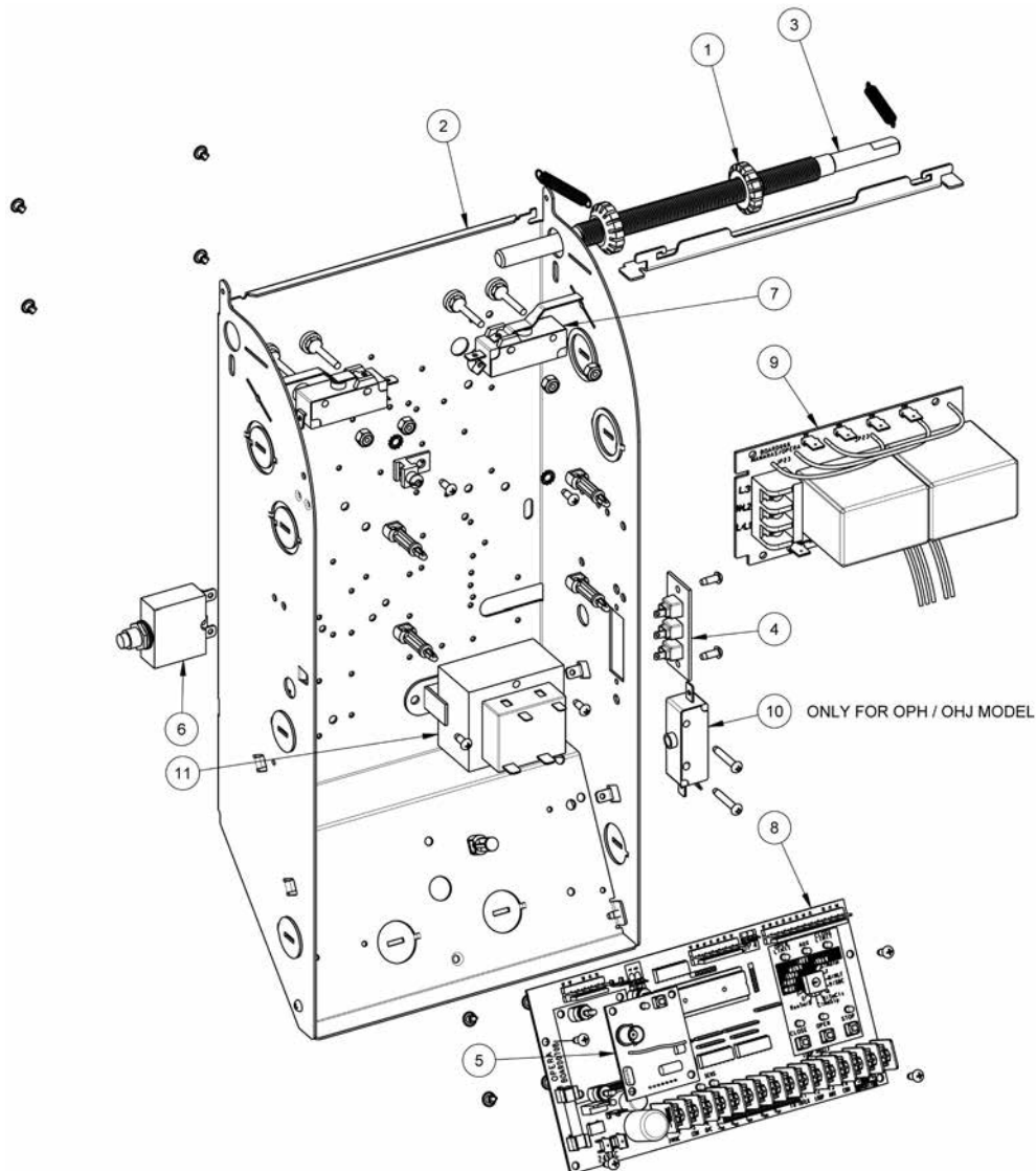
Figura 53 - Caja de control Opera con tablero de control electrónico BOARD070M/E
