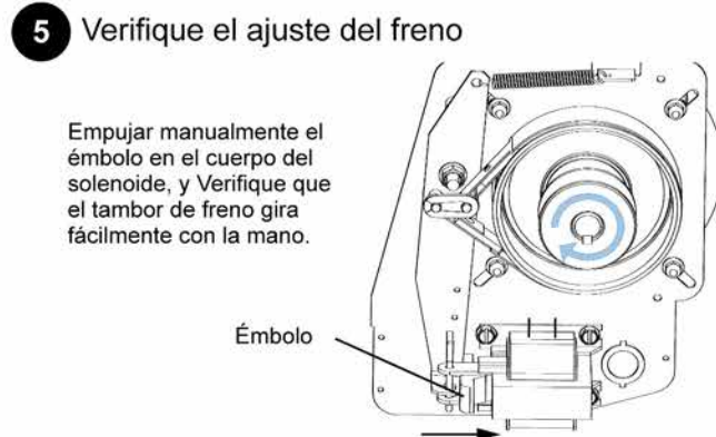
Figura 43 - Procedimiento de ajuste de la banda de freno
