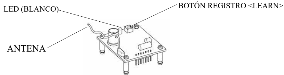
Figura 40 - RADIORE100 (ECB BOARD 070)
