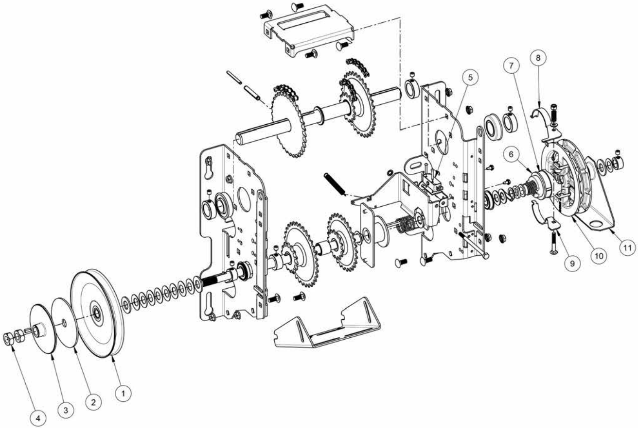
Figura 50 - Despiece mecánico Opera-HJ
