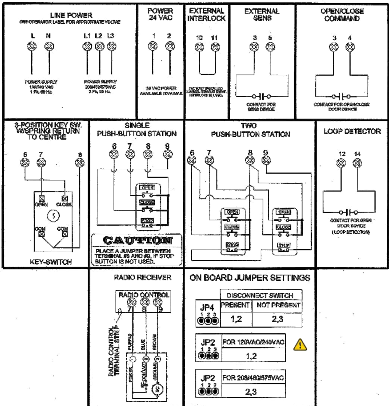
Figura 22 - Cableado externo
