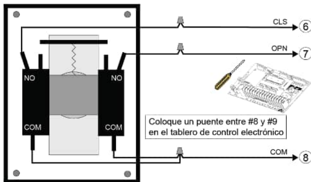
Figura 19 - KEYSWITCH 010 / 015 (Interruptor de llave)
