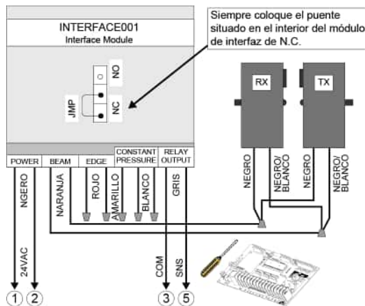
Figura 8 - PHOTO 008C3 / C4 / E1 (celdas fotoeléctricas)
