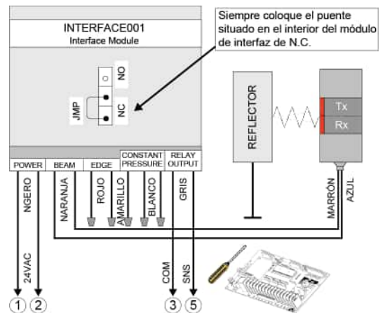
Figura 9 - PHOTO 008D1 / D2 (celdas fotoeléctricas)
