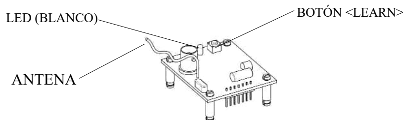
Figura 24 - RADIORE100 (ECB BOARD 070)
