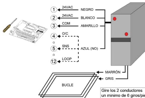
Figura 21 - Detector de bucle de vehículo
