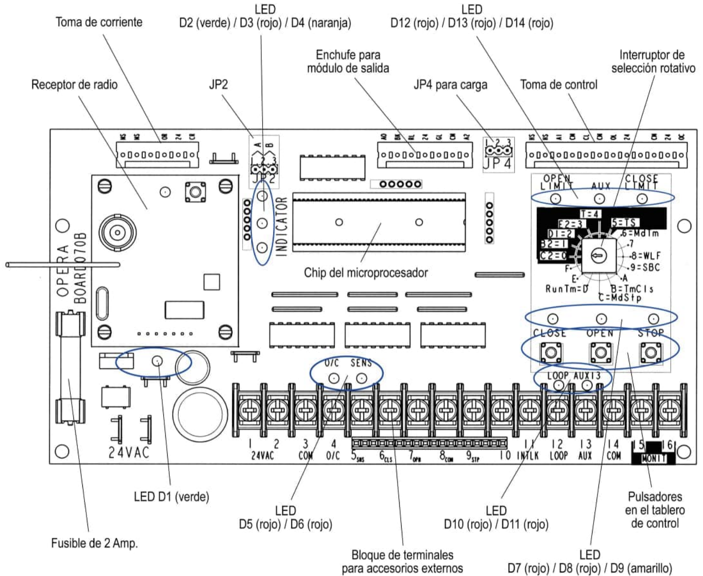
Figura 23 - Tablero de control electrónico – BOARD 070E
